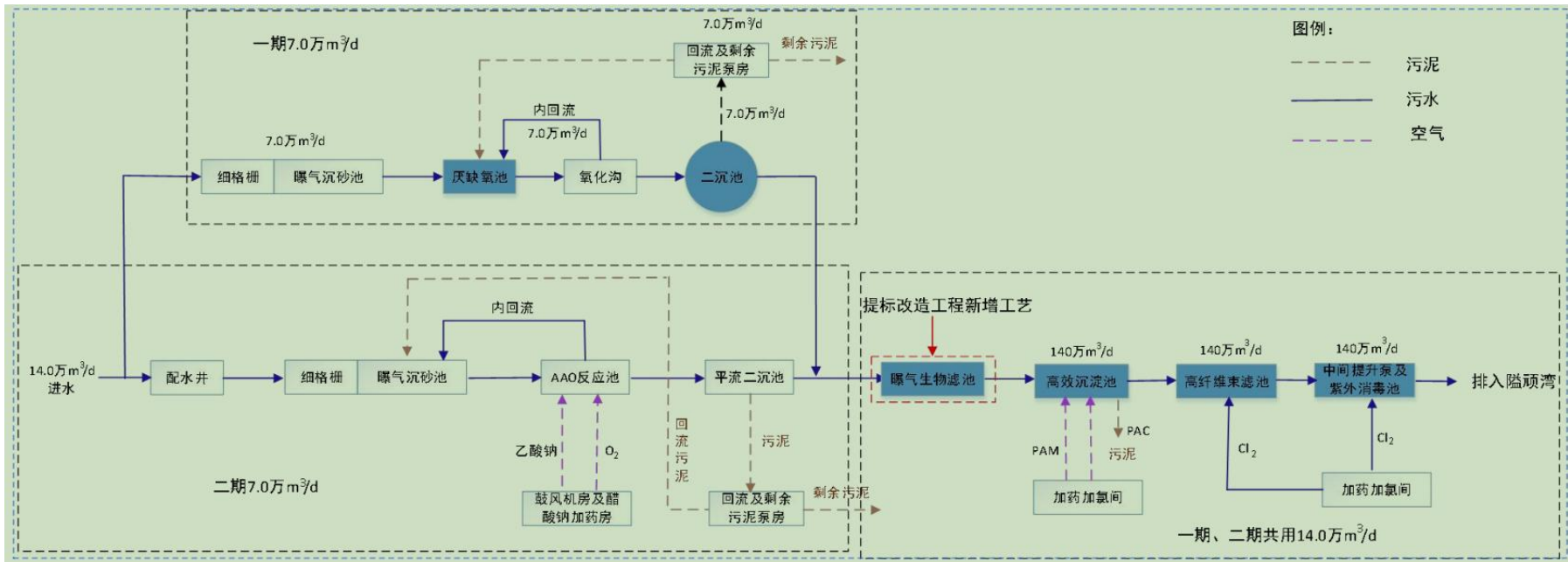
图 4-1 温岭市观岙污水处理厂工艺流程
