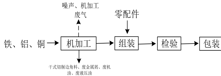
图 2-2 项目喷涂机生产工艺流程图
