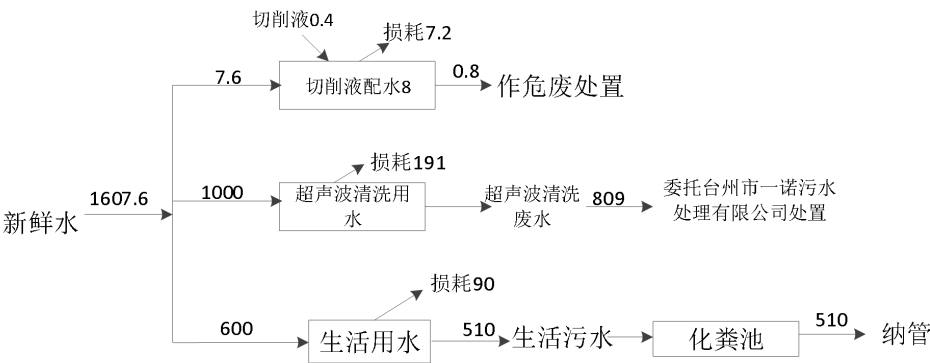
图 2-1 水平衡图 (t/a)
