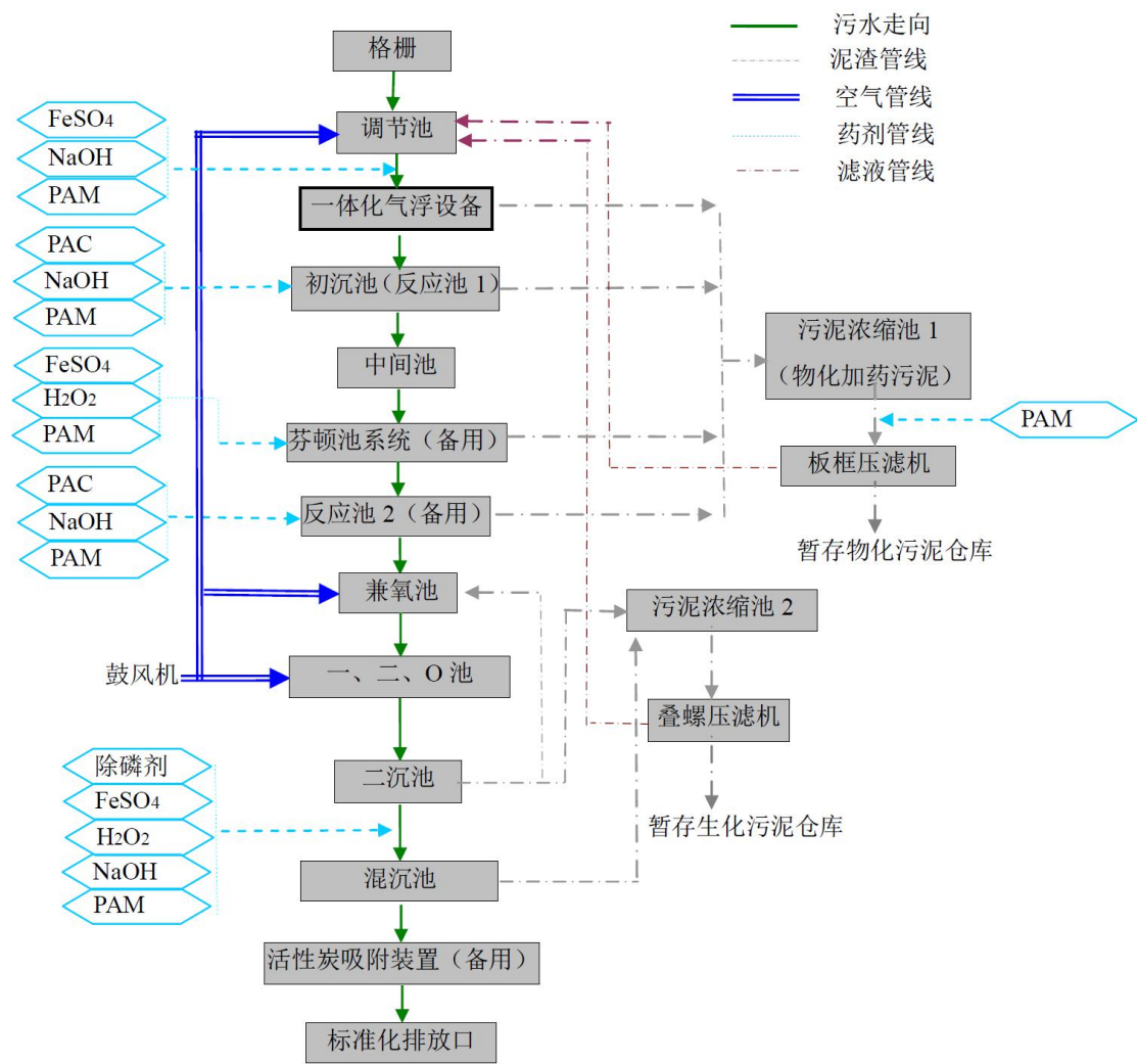
图 4-2 污水处理工艺流程图
